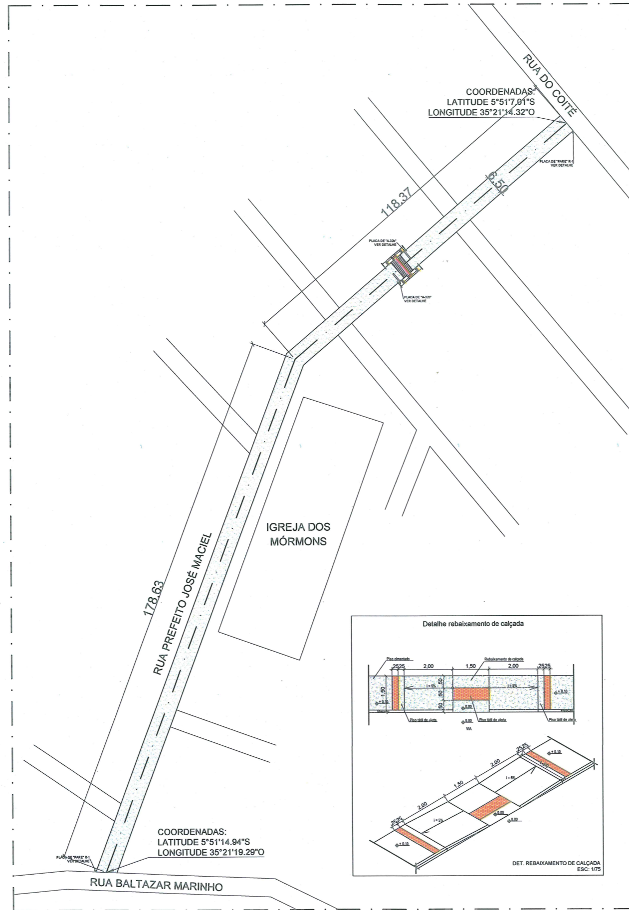
PLANTA SITUAÇÃO E LOCAÇÃO ESC.: 1/600
