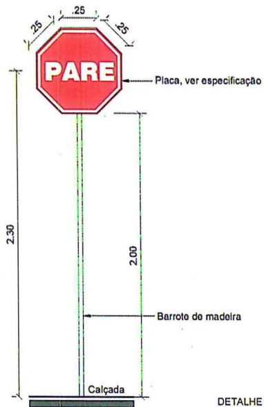
DETALHE 01 ESC: 1/25
