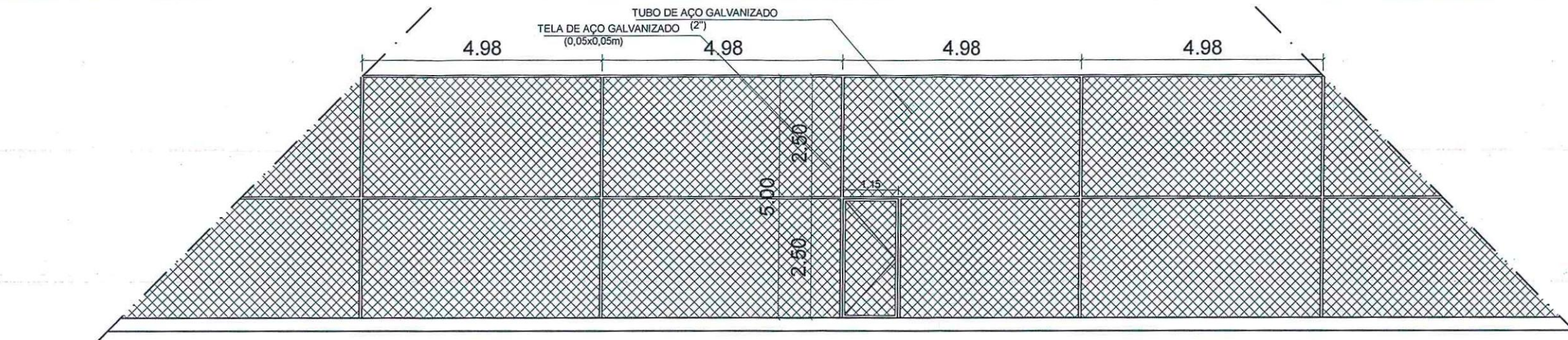
VISTA FRONTAL ALAMBRADO ESC.: 1/100
