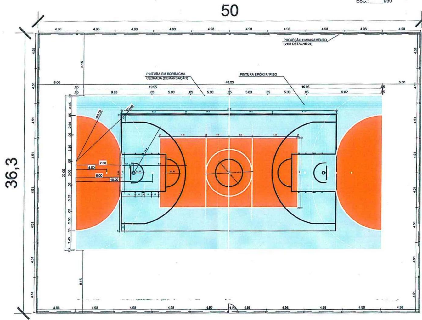
PLANTA BAIXA ESC.: 1/300
