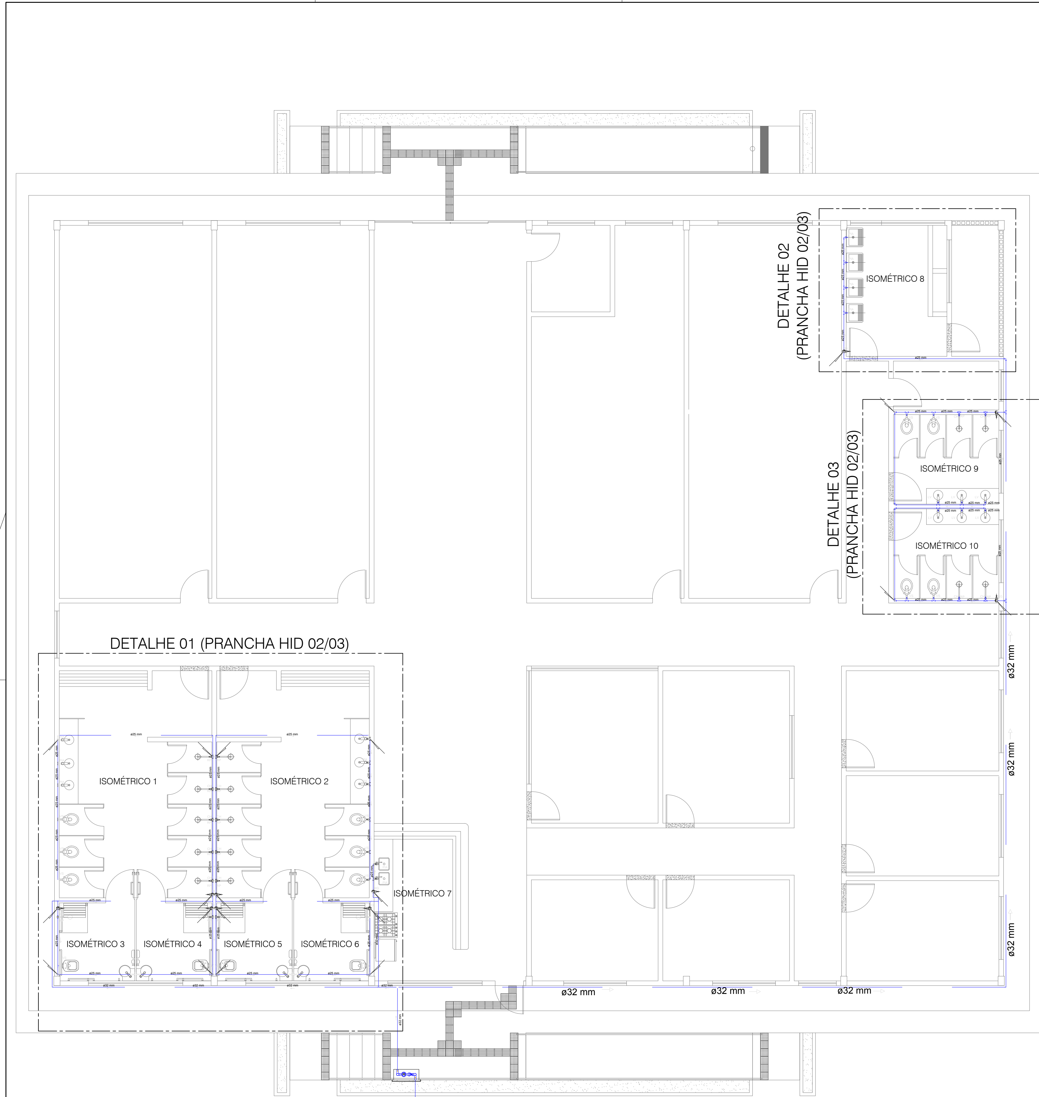
PLANTA BAIXA DE IMPLANTAÇÃO ESC. 1:75
