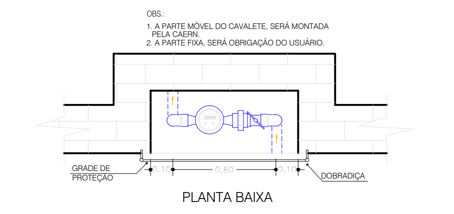
DETALHE DE ABRIGO P/ HIDRÔMETRO SEM ESCALA
