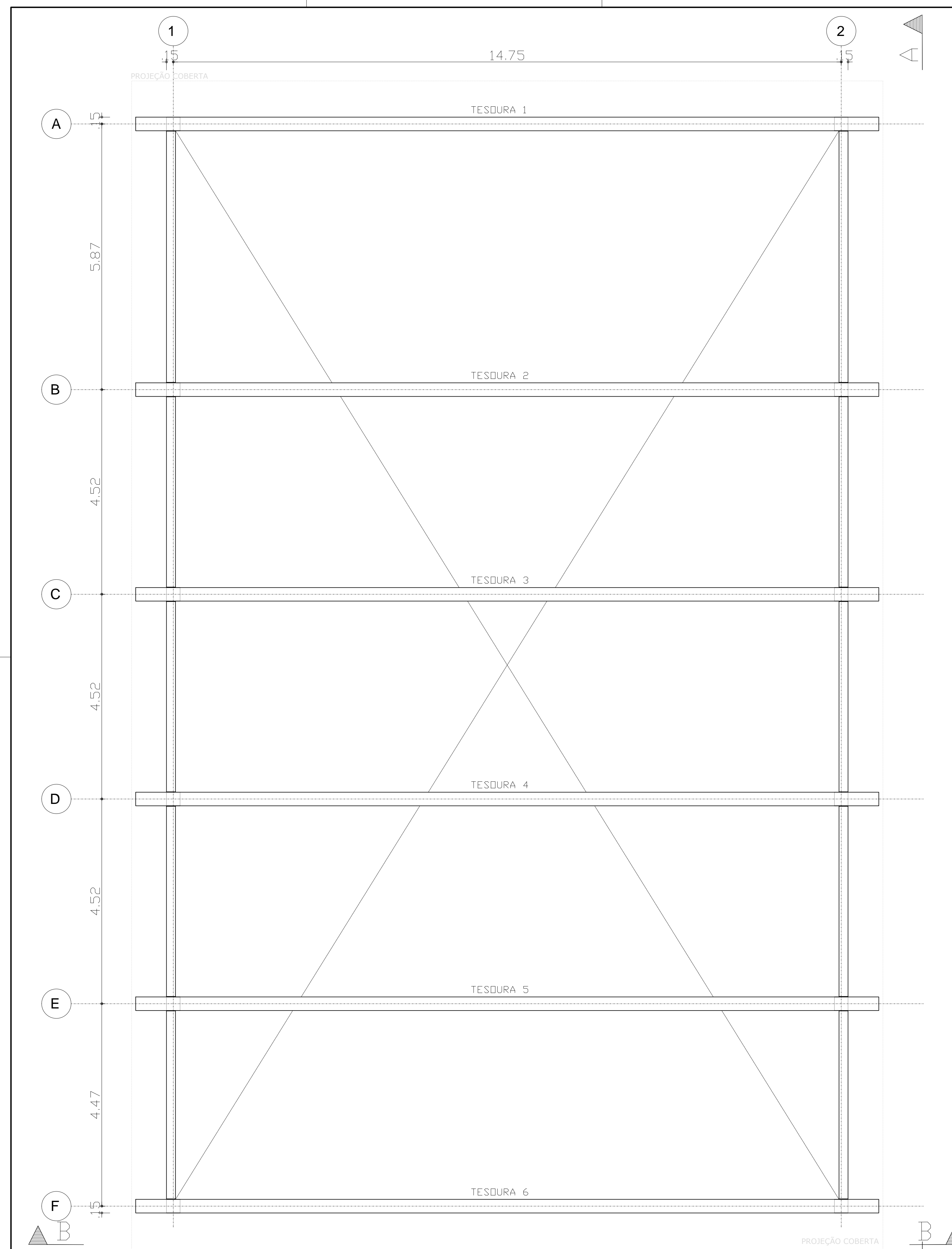
FORMA DA COBERTURA - (NÍVEL 2) ESCALA 1:50
