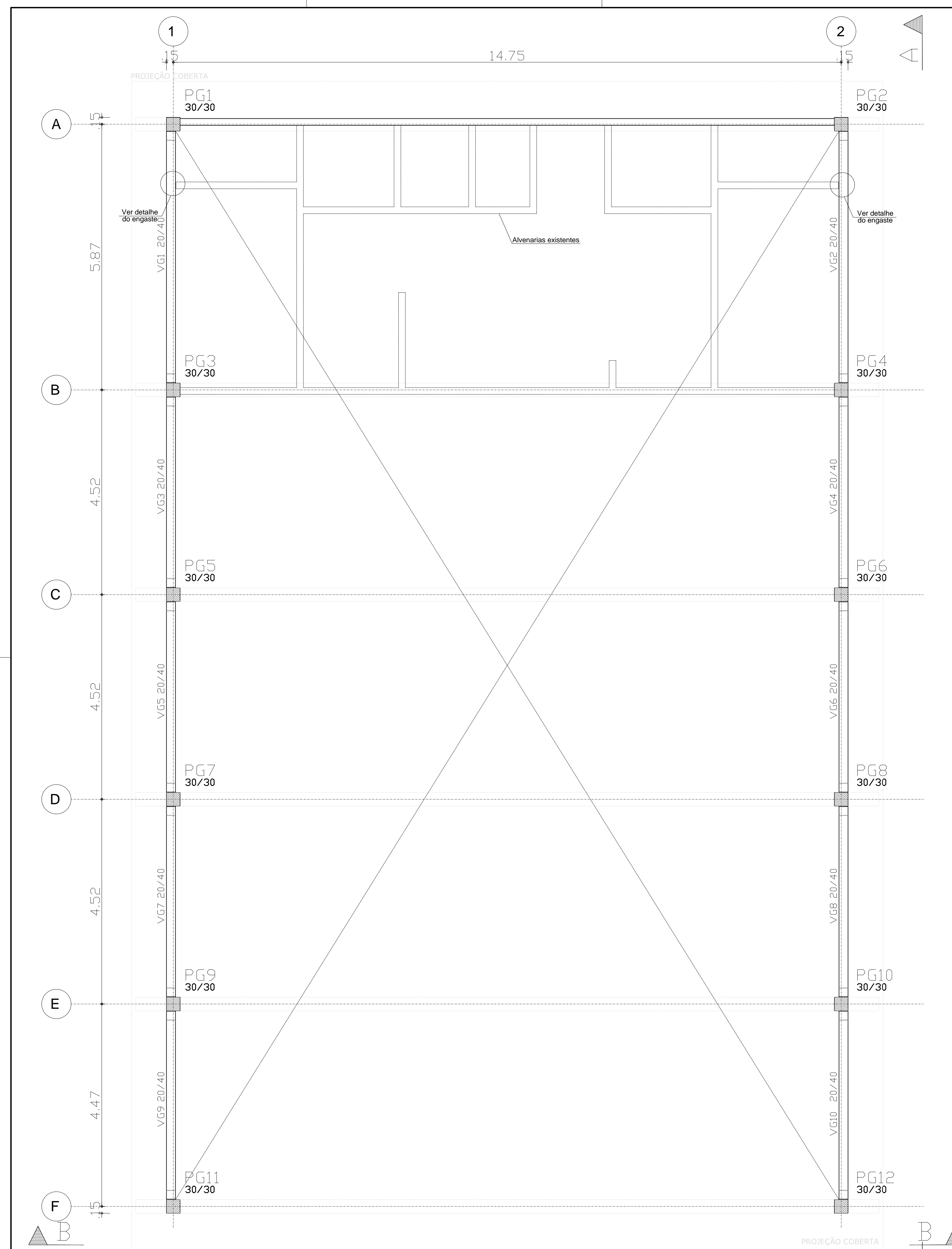
FORMA DA COBERTURA - (NÍVEL 1) ESCALA 1:50
